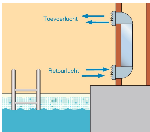
Inbouwmodel SBA...P
